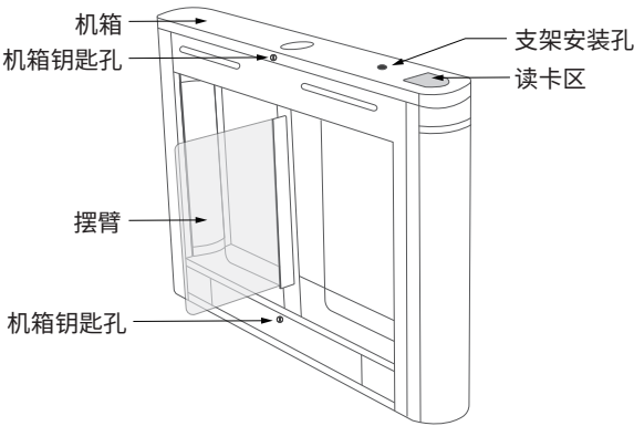
图1-1 外部结构图
