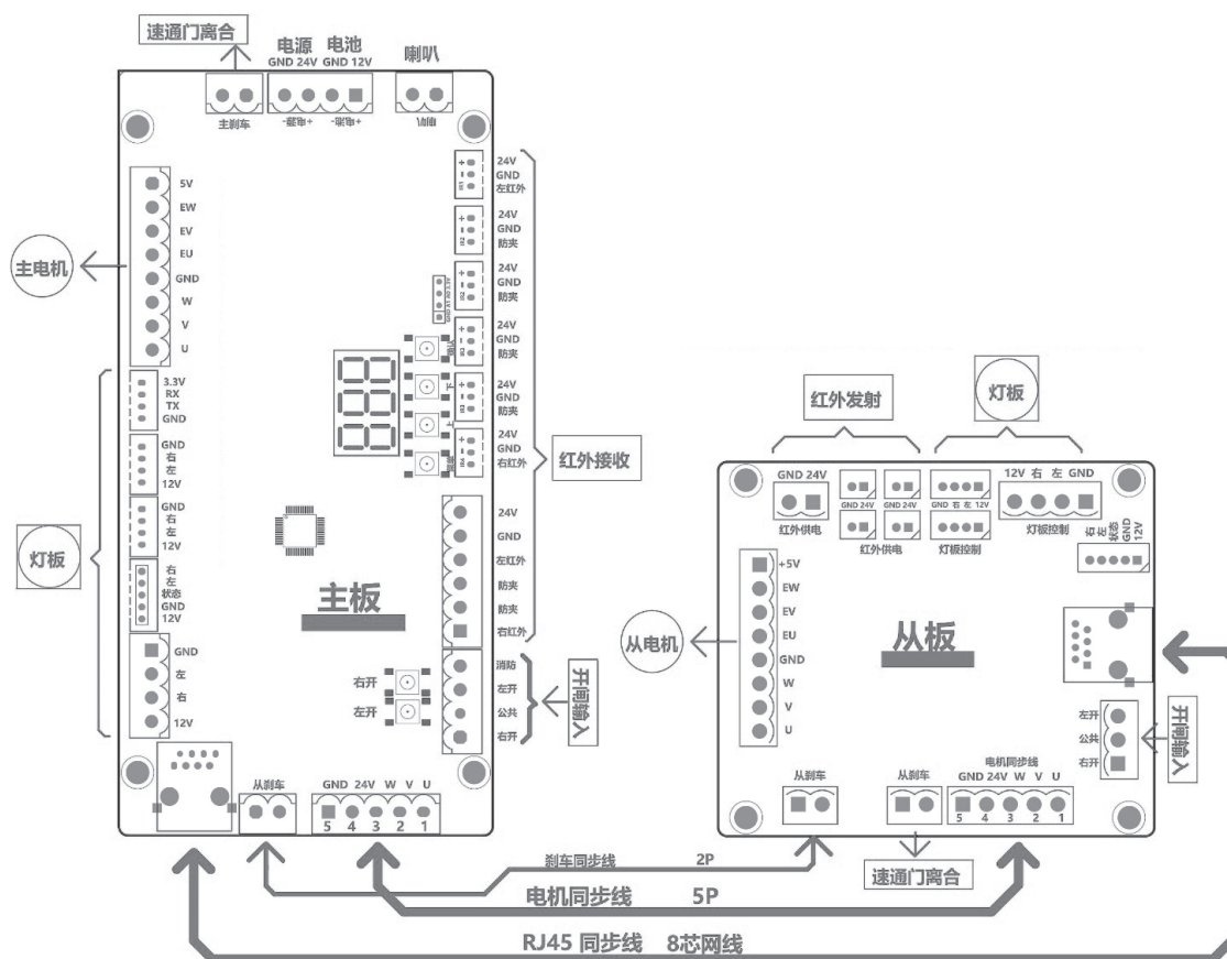
图3-1 控制主板接口描述图
