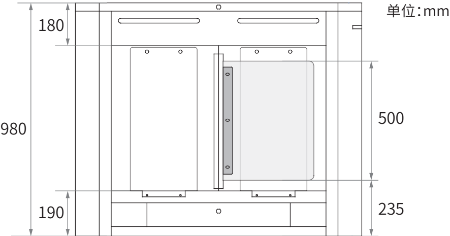
图1-3 道闸侧视图
