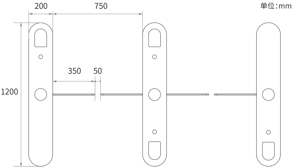
图1-2 道闸俯视图
